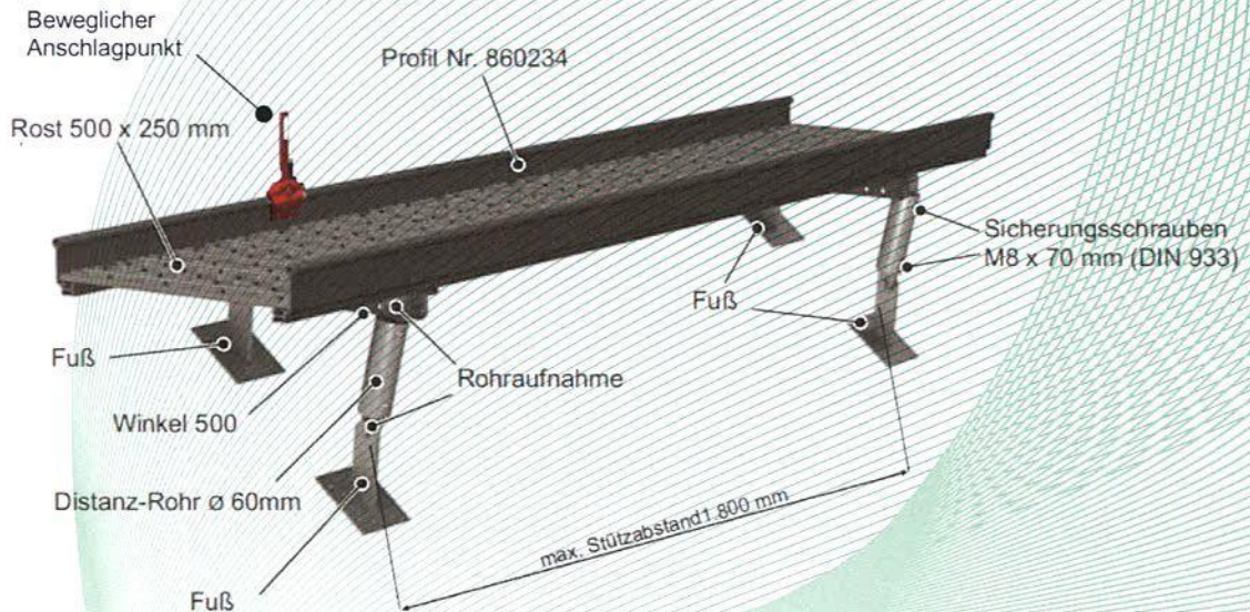
Bild 1: Laufsteg Typ C – Klasse 2 (K2), Typ: Wartungsweg Typ C, montiert auf Schiefer
