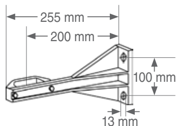
Wandanker
