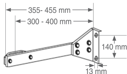
Wandanker (Alu-Profil)
